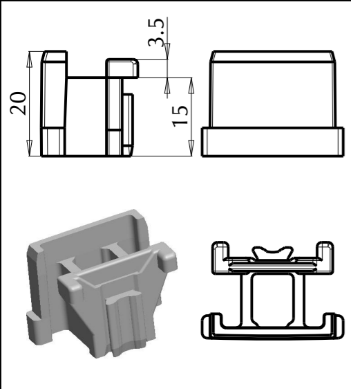
STAFFA U52 QUADRA x ART.300 N°0 CODICE: STFR1900N060 COLORE: NERO
