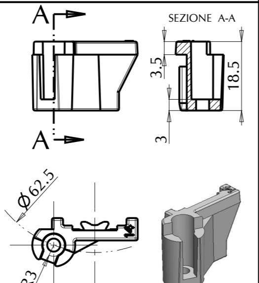
STAFFA U52 INTERASSE 62.5 N°14 CODICE: STFR1900D140 COLORE: BIANCO
