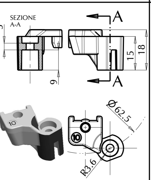
STAFFA U52 INTERASSE 62,5 N°10 CODICE: STFR1900D100 COLORE: BIANCO
