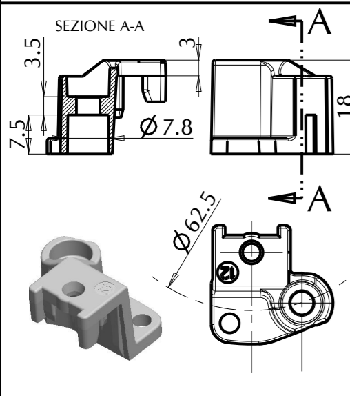
STAFFA U52 INTERASSE 62,5 N°12 CODICE: STFR1900D120 COLORE:
